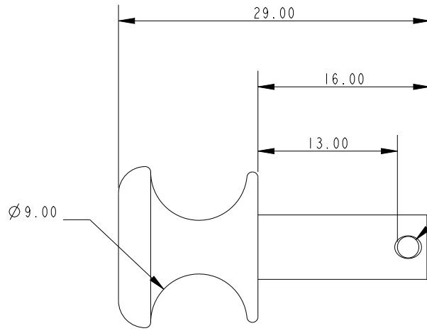
SCALE 2:1
